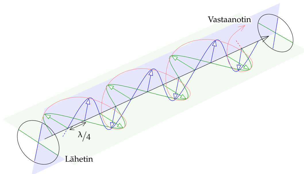
KUVA 7.4. Ympyräpolarisoidut radioaallot kulkevat lähettimestä vastaanottiin. Ympyräpolarisoitu aalto saadaan yhdistämällä kaksi aaltoa, jotka ovat lineaarisesti polarisoituja keskenään kohtisuorissa suunnissa, ja joiden välillä on vaihesiirtymä \pi/2 .
