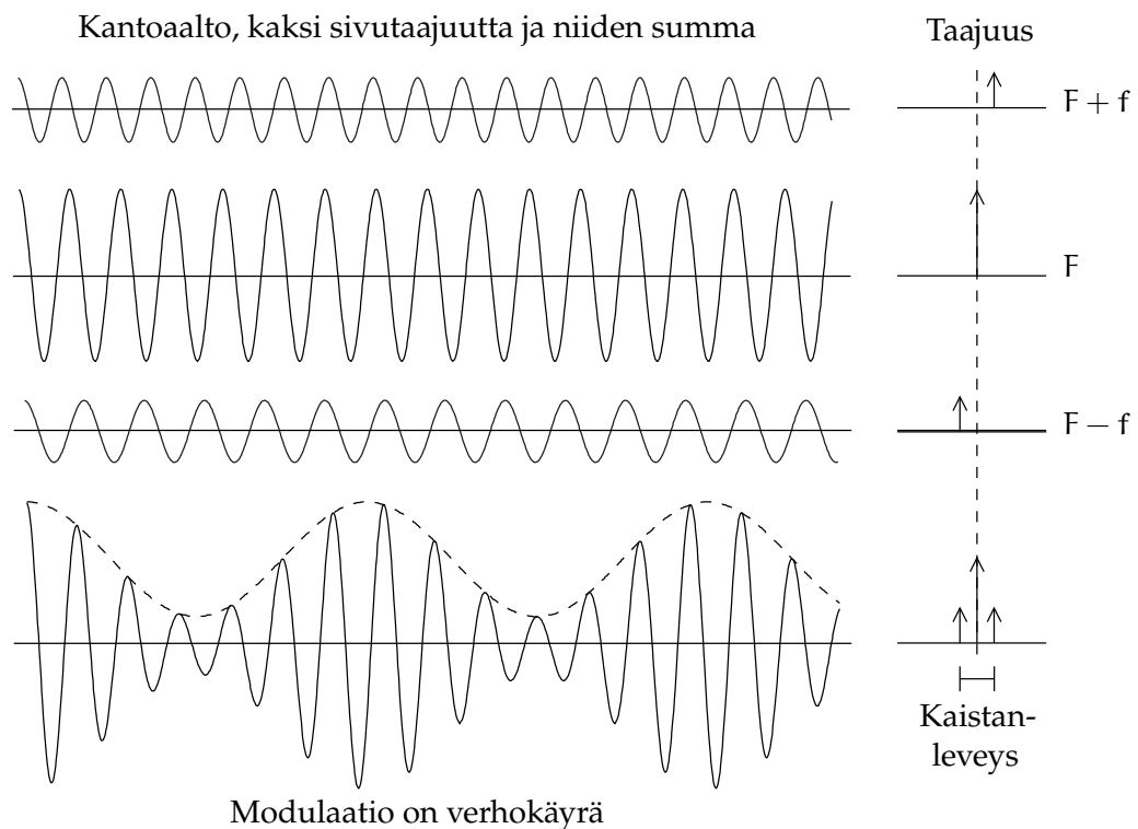
KUVA D.1. Amplitudimodulaatio ja kaistanleveys.
