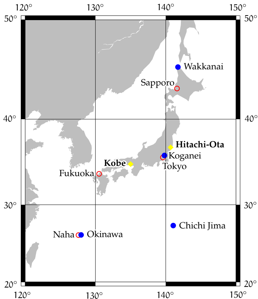
KUVA 10.4. MSASin ja QZSSin maalohko, tilanne noin vuonna 2016. Keltainen: Master Control Station (MCS). Ground Monitor Station (GMS), punainen: MSAS, sininen: QZSS.
