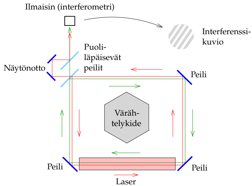
KUVA 5.7. Sagnacin interferometriin perustuva rengaslasergyroskooppi.
