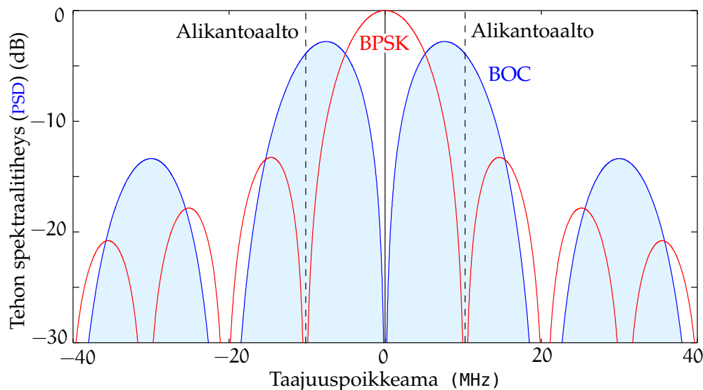
KUVA 7.14. Esimerkki siitä, miten BOC siirtää tehoa sivukaistoihin.
