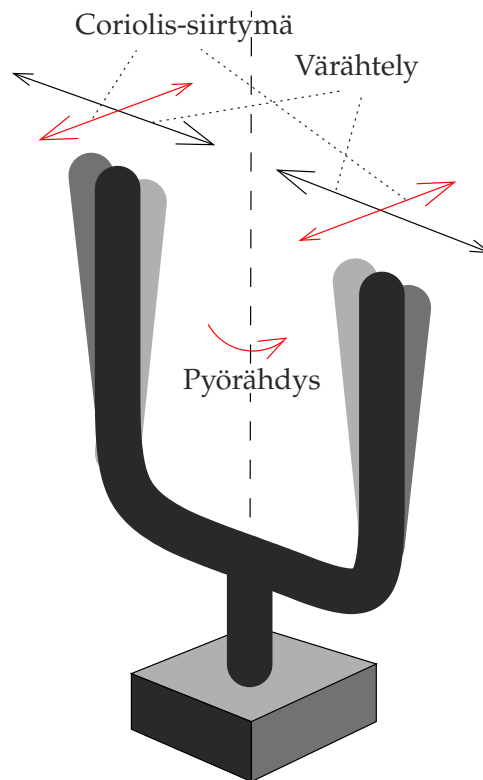
KUVA 13.4. MEMS-pyörähdysanturin periaate. Jos alusta pyörii, aiheuttaa ääniraudan värähtely (kuvassa vasen-oikea) coriolisvoiman kautta jaksollisen siirtymän, joka mitataan kapasitiivisesti.
