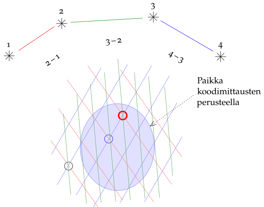
KUVA 9.1. Kokonaislukutuntemattomien ratkaisu. Tässä kuvassa viivakimput (punaiset, vihreät ja siniset) edustavat liikkuvan vastaanottimen mahdollisia paikkoja, jotka ovat yhteensopivia havaittujen vaiheen kaksoiserotusten kanssa. Kokonaislukutuntemattomien ratkaisun on oltava yhteensopiva kaikkien havaittujen kaksoiserotusten kanssa (punainen ympyrä), mutta myös kontrastin toiseksi parhaiten sopivan ratkaisun (sinisen ympyrän) kanssa on oltava selkeä.
