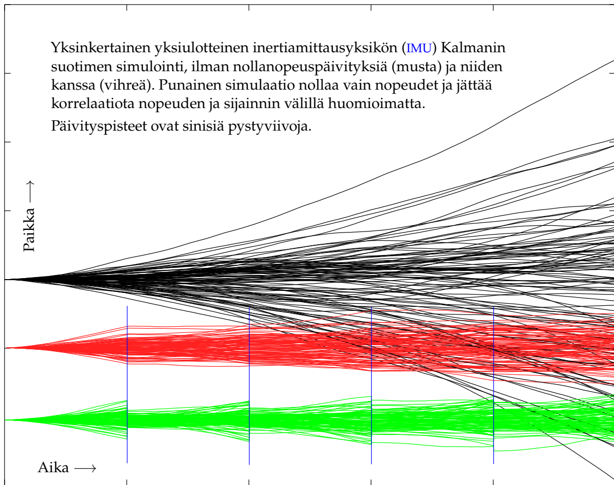
KUVA 13.2. Yksinkertainen Kalmanin suodin ilman nollanopeuspäivityksiä ja niiden kanssa.
