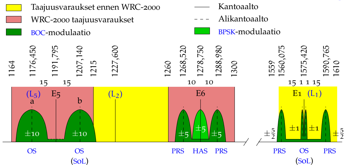
KUVA 11.2. Galileon taajuudet ja modulaatiot, yksikkö MHz. WRC-2000 oli World Radiocommunications Conference Istanbulissa vuonna 2000. Kuvassa on tyylitelty kuvio, jossa vihreiden alueiden (päähuippujen) puolileveydet edustavat koodien bittinopeuksia. Taajuserot ja -hajonnat ovat "GPS-megahertseinä", jotka ovat 1,023 MHz:n kokoisia.
