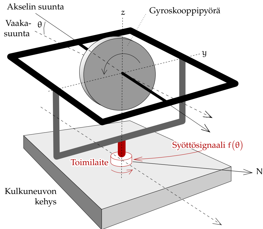
KUVA 5.9. Vakautetun alustan periaate. Syöttösignaali aiheuttaa prekessioliikkeen, joka pitää gyroskoopin akselin suunnan vaakatasossa. Tavallisesti pystysuoraa akselia eli z-akselia, jonka ympäri kohdistuu vääntöä, kutsutaan syöttöakseliksi ja vaakasuoraa y-akselia, jonka ympäri syntyy prekessiota, lähtöakseliksi.
