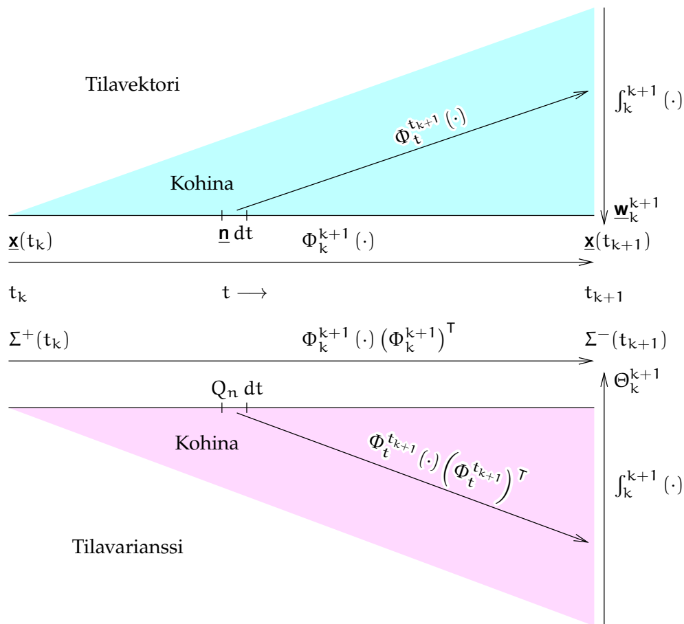
KUVA 3.3. Tilavektorin ja tilavarianssin eteneminen kohinan läsnä ollessa.
