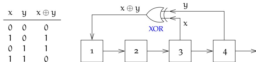
KUVA 7.9. Lineaarisen palautteen siirtorekisteri. Vasemmalla XOR-operaation määritelmä.
