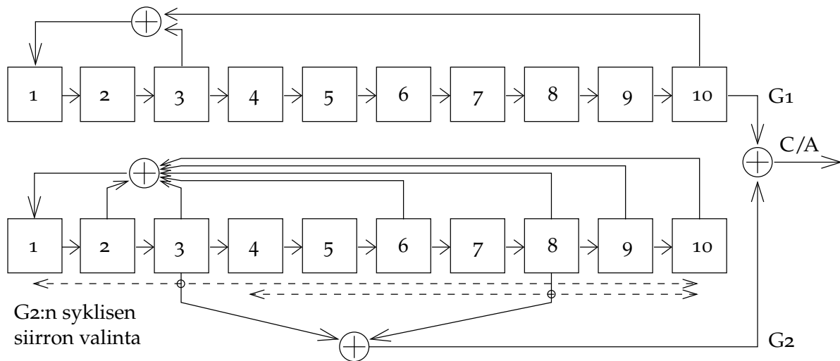
KUVA B.1. C/A-koodin muodostaminen käyttämällä kahta kymmenen solun lineaarisen palauteen siirtorekisteriä G1 ja G2, joiden palautehanojen geometriat ovat erilaisia. Rekisterin G2 syklinen siirto rekisterin G1 suhteen, joka on erilainen jokaiselle satelliitille, asetetaan ennen laukaisua valitsemalla ja sekoittamalla kaksi solulähtöä: y^\alpha \oplus y^{\alpha'} \rightarrow y^\beta . Paikkojen 3 ja 8 valitseminen, kuten kuvassa, tuottaa PRN-koodin 31.
