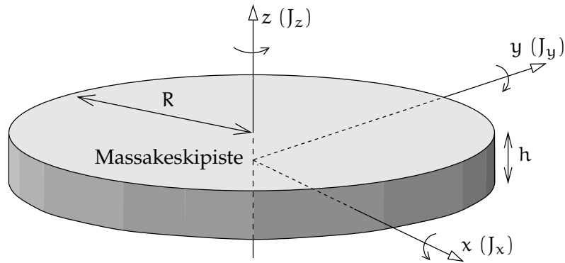
KUVA 5.3. Gyroskoopin roottori ja sen päähitausmomentit.
