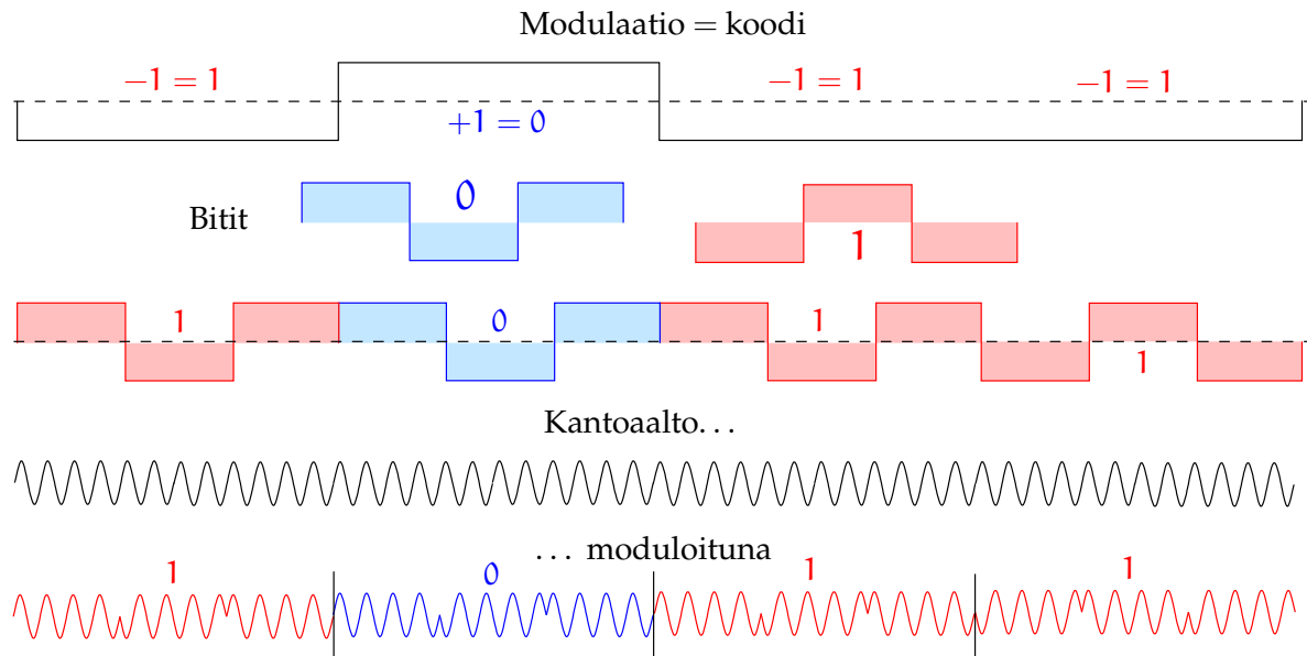
KUVA 7.13. BOC, binaarinen offset kantaaltomodulaatio. Esimerkki.
