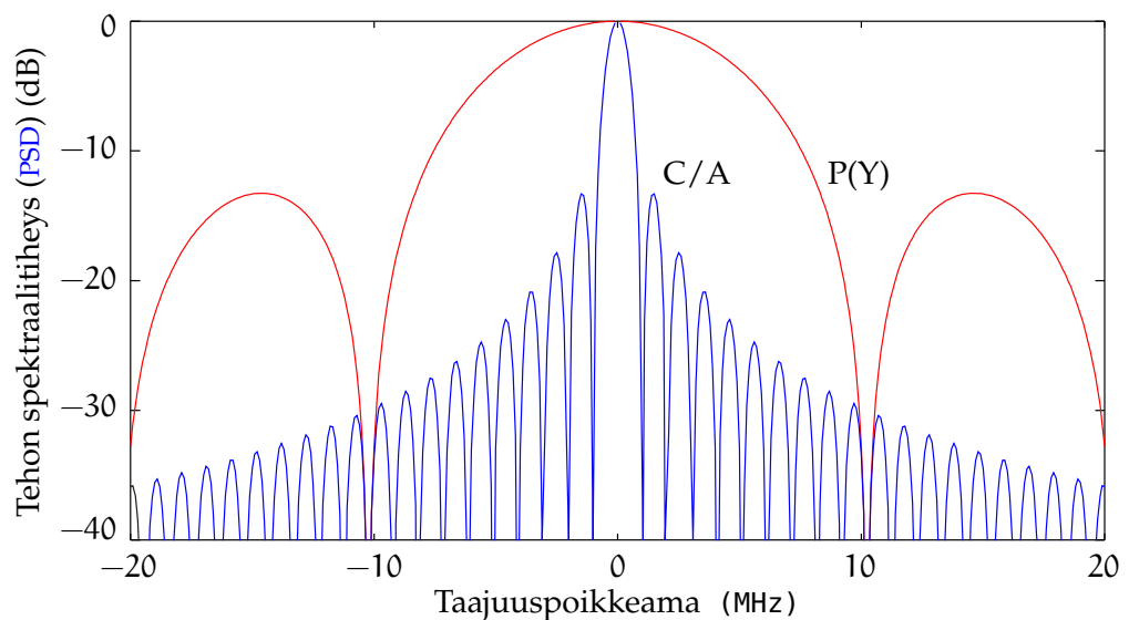
KUVA 7.12. Alkuperäisen GPS-signaalin tehospektri.
