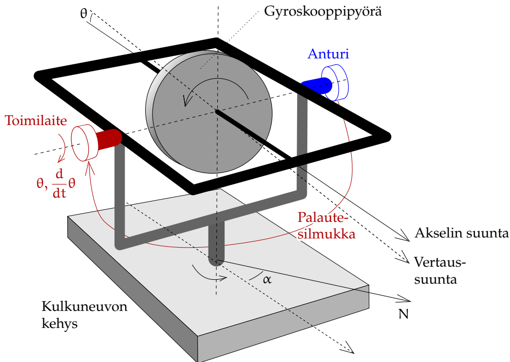
Kuva 5.10. Hyrräkompassin periaate. Palautesilmukka tuottaa prekessioliikkeen, joka saa gyron pyörimisakselin kääntymään pohjoiseen.
