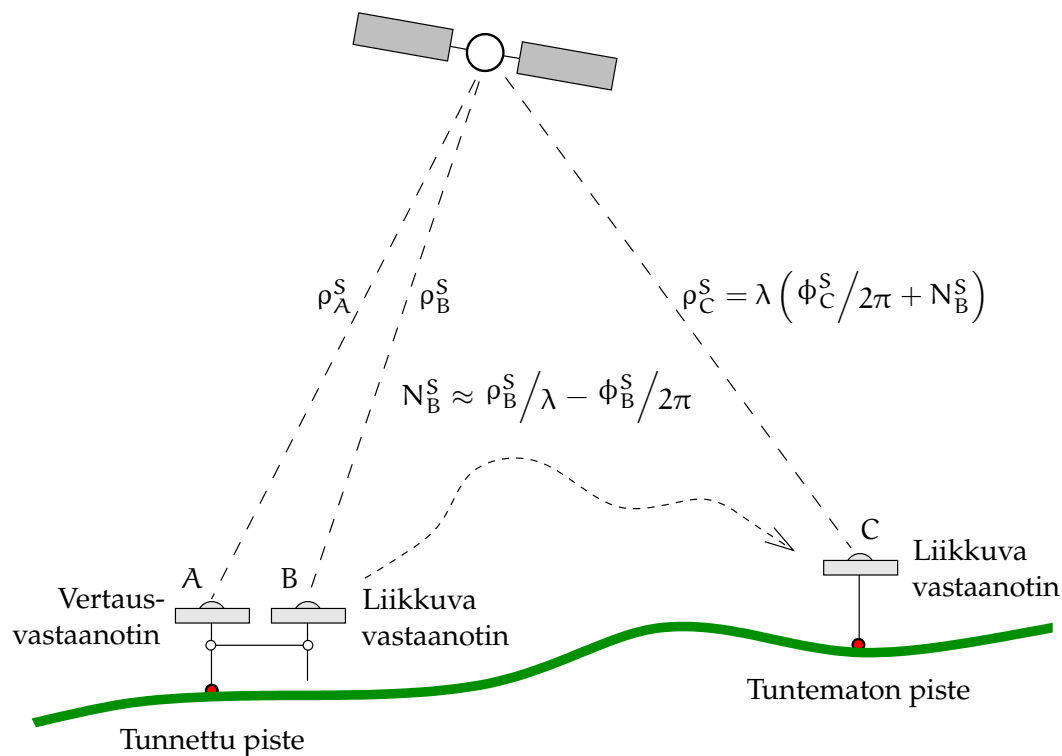
Kuva 8.3. Tosi aikaisen kinemaattisen GNSS-paikannuksen idea. Ko-lokaation avulla voidaan määrittää kokonaislukutuntematon N , mikä mahdollistaa satelliitin todellisen etäisyyden määrittämisen tuntemattomalla paikalla C. Oletettu on tässä, epärealistisesti, että kaikki mitatun kanta-aallon vaiheen \phi muutokset ovat satelliitin ja vastaanottimen välisen geometrisen etäisyyden \rho muutosten aiheuttamia.
