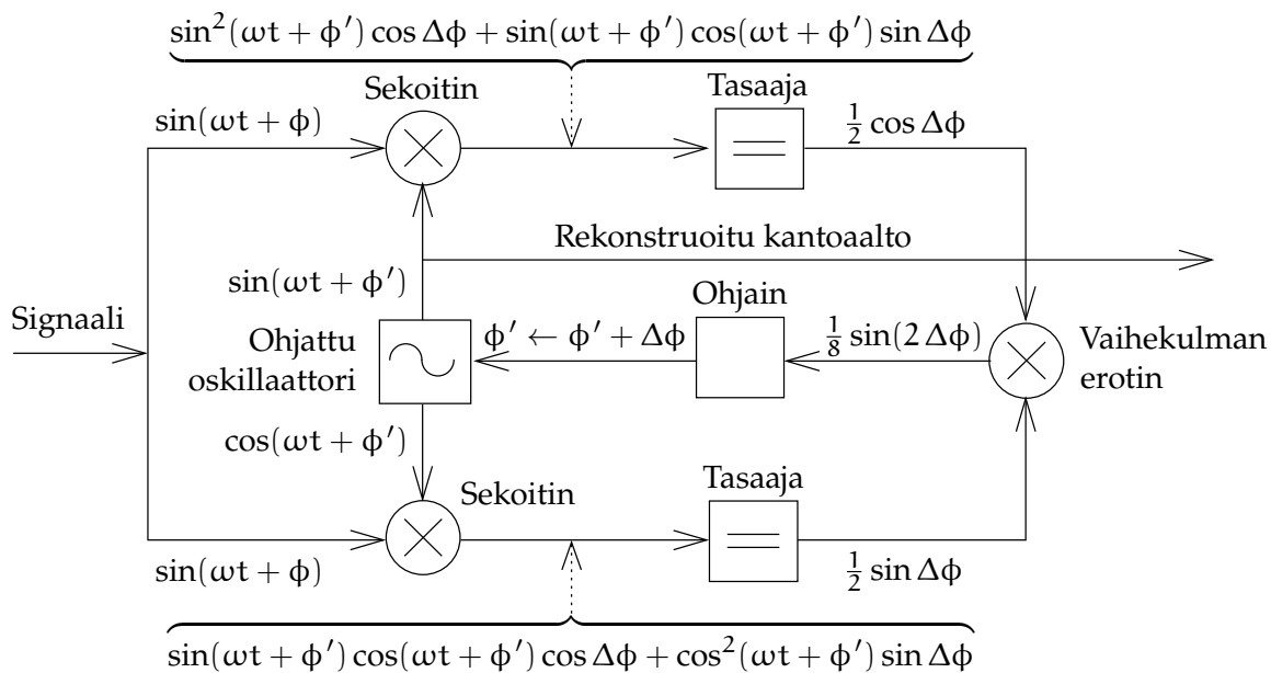
KUVA 7.16. Costasin diskriminaattorin eli silmukan suorittama kanta-aallon vaiheen seuranta.
