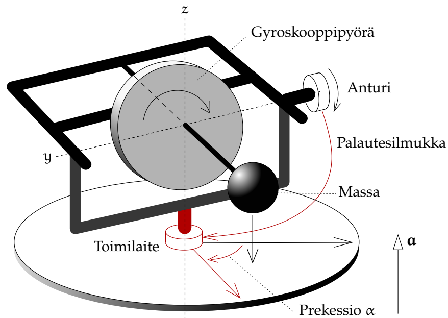
Kuva 5.6. Gyroskooppipohjainen heilurikihtyvyyssmittari. Kulma \alpha on kokonaisprekessiokulma, joka on verrannollinen mitatun kiihtyvyyden aikaintegraaliin.
