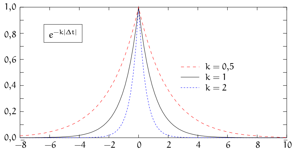
KUVA 2.4. Stationaarisen Gaussin ja Markovin prosessin autokovarianssifunktio aikaeron \Delta t = t - t' funktiona. Oletettu on A_x(0) = Q_n/2k = 1 .
