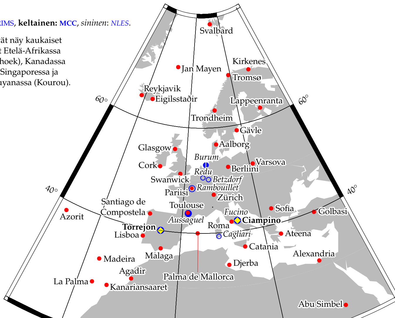
Kuva 10.3. EGNOSin maalohko, tilanne 2019.
