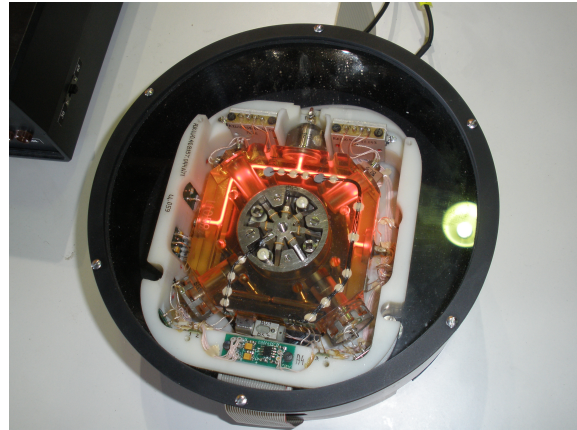
KUVA 5.1. Vasemmalla gyroskooppi. Wikimedia Commons, Gyroskooppi . Nap-sauta animaatiota varten. Oikealla ilmailussa käytetty rengaslaser-gyroskooppi. Nockson (2011) .
