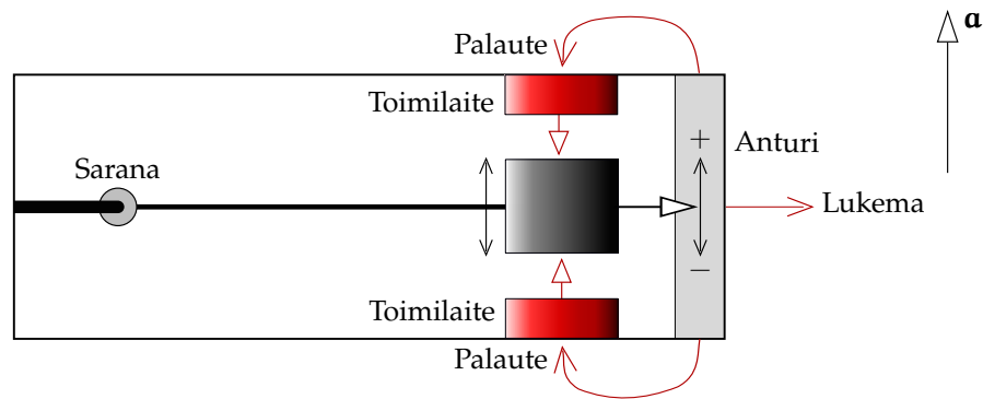
Kuva 5.5. Heilurikihtyvyyssmittari.
