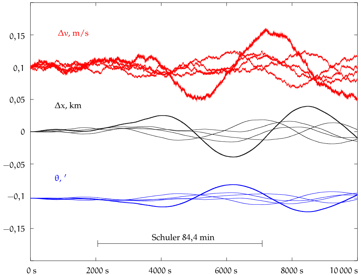
KUVA 5.13. Virheiden kasautuminen yhtälön 5.27 yksiulotteisen mekanisoinnin mukaan. Käytetyt arvot ovat: \underline{n}_a on \pm 100 mGal, \underline{n}_g = 0 . \Delta v - ja \theta -käyrät on siirretty selkeyden vuoksi.
