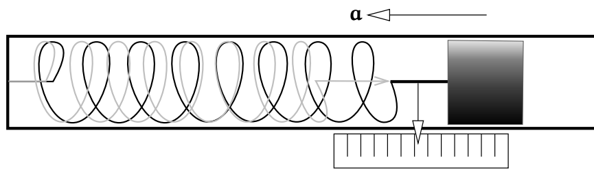
KUVA 5.4. Jousikiihtyvyyssmittarin periaate.
