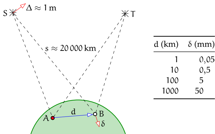
KUVA 8.2. Differentiaalipaikannuksen tarkkuuden arvioimisen geometria. Oletettu ratavirhe \Delta = 1 m vastaa broadcast ephemeris -rataennusteiden nykyistä tarkkuutta.
