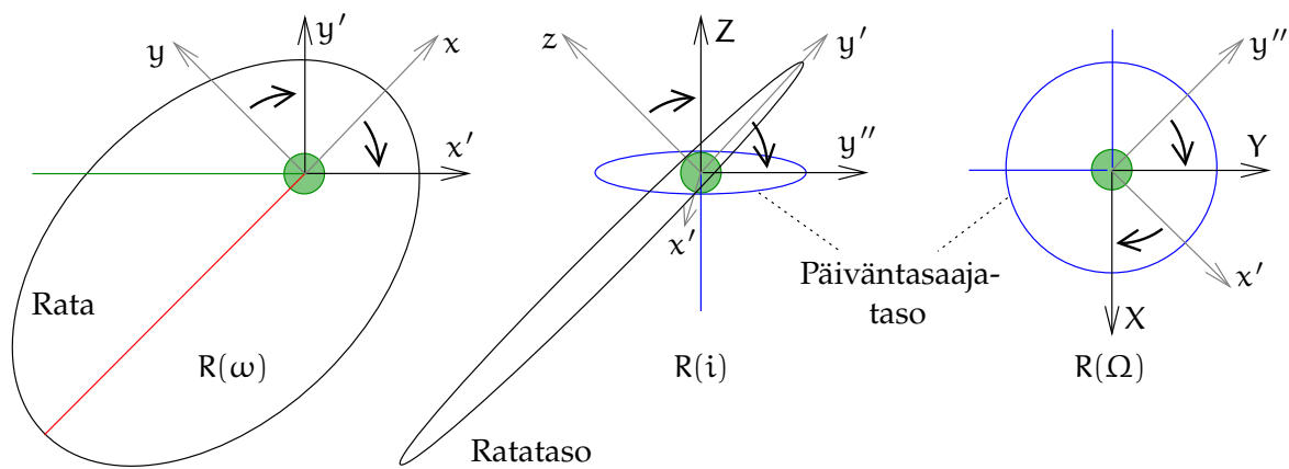
KUVA 6.4. R-matriisin johtaminen.
