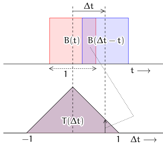
KUVA 7.11. GPS-modulaation autokovarianssifunktio.
