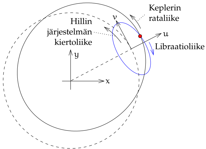
Kuva 6.6. Libraatioliike.
