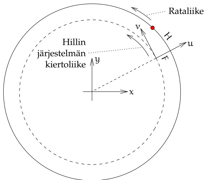
Kuva 6.7. Lineaarinen ajelehtiminen, jos satelliitin periodi eroaa Hillin koordinaatiston periodista.
