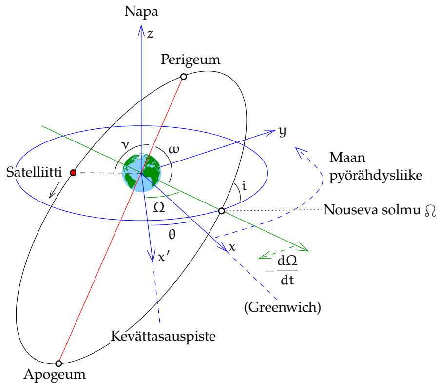
KUVA 6.1. Keplerin rata-alkiot avaruudessa.
