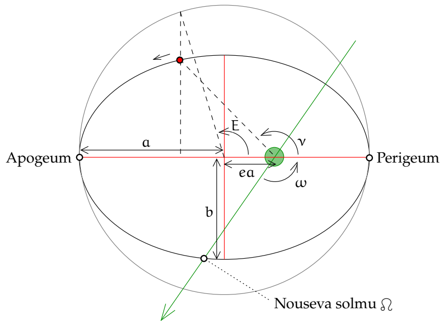
Kuva 6.2. Keplerin rata-alkiot tasossa.
