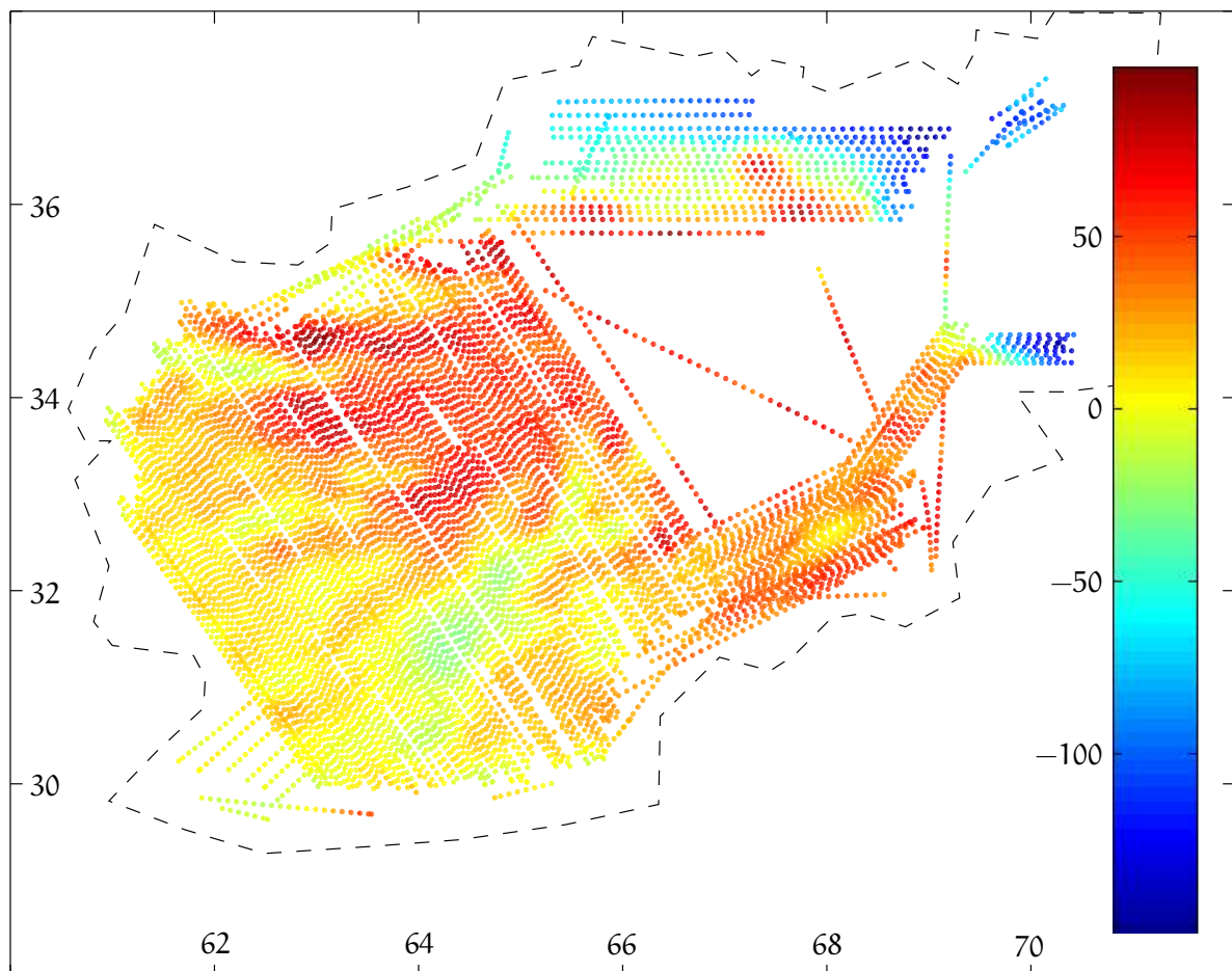
KUVA 12.2. Afganistanin ilmagravimetriakartoitus. Värät esittävät ilma-anomaliaita lentokorkeudella. Yksikkö on milligal ( USGS Open-File Report 2008-1089 ). Alkuperäisaineistoa on harvennettu 50×.
