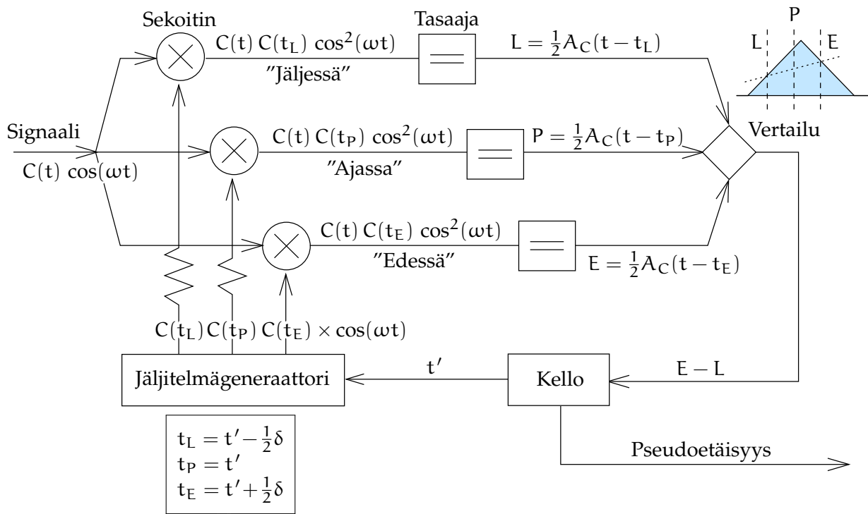
KUVA 7.15. GPS-koodiseuranta.
