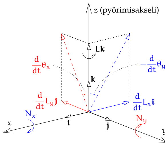
Kuva 5.2. Kuinka vääntö aiheuttaa gyroskoopin pyörimisakselin prekessiota. Huomaa korkkiruuvivääntö: N_x , N_y , \frac{d}{dt} L_x , \frac{d}{dt} L_y ja \frac{d}{dt} \theta_y ovat negatiivisia ja L ja \frac{d}{dt} \theta_x ovat positiivisia.
