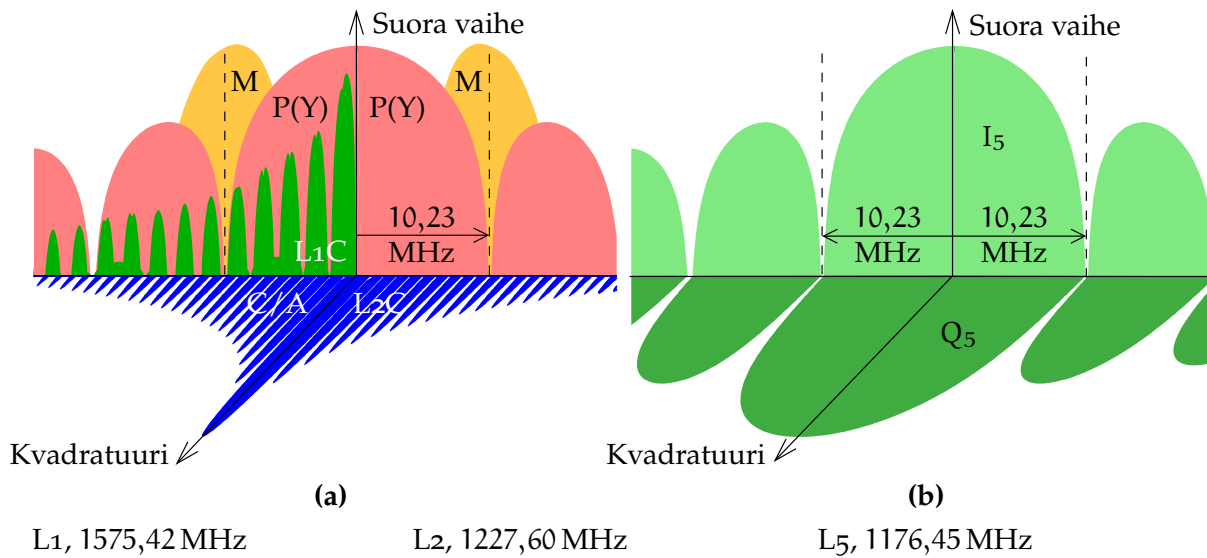
KUVA 7.3. Kantoaallon suoran vaiheen ja kvadratuurin vaihekuilmiöiden GPS-koodien tehospektrit. L1 ja L2 annetaan yhdistetyssä kuvassa: C/A ja L1C moduloidaan taajuudelle L1, kun taas L2C moduloidaan samalla tavalla taajuudelle L2.
