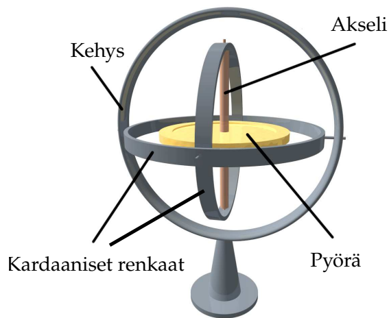
KUVA 5.1. Vasemmalla gyroskooppi. Wikimedia Commons, Gyroskooppi . Nap-sauta animaatiota varten. Oikealla ilmailussa käytetty rengaslaser-gyroskooppi. Nockson (2011) .
